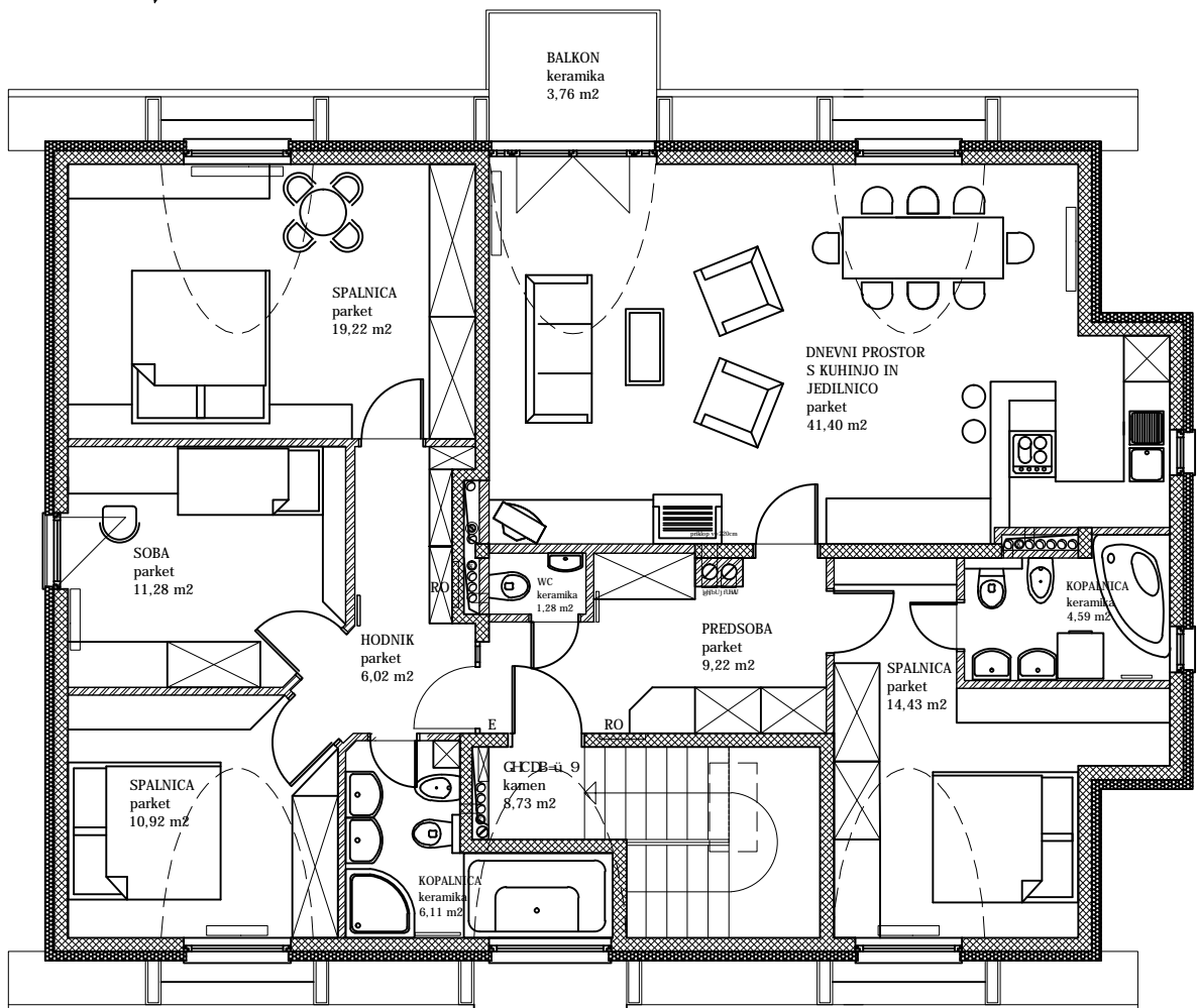
MANSARDA objekt B M 1:100
