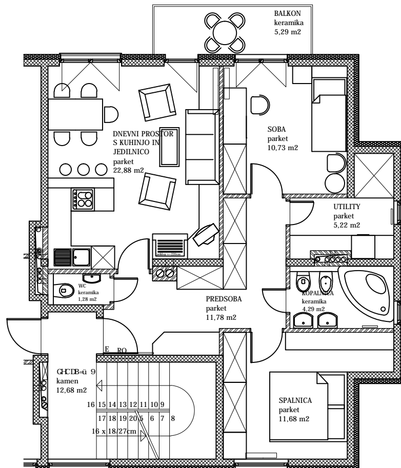
NADSTROPJE objekt B M 1:100
