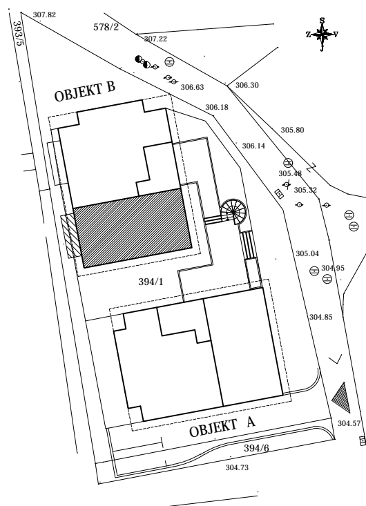
SITUACIJA M 1:500
