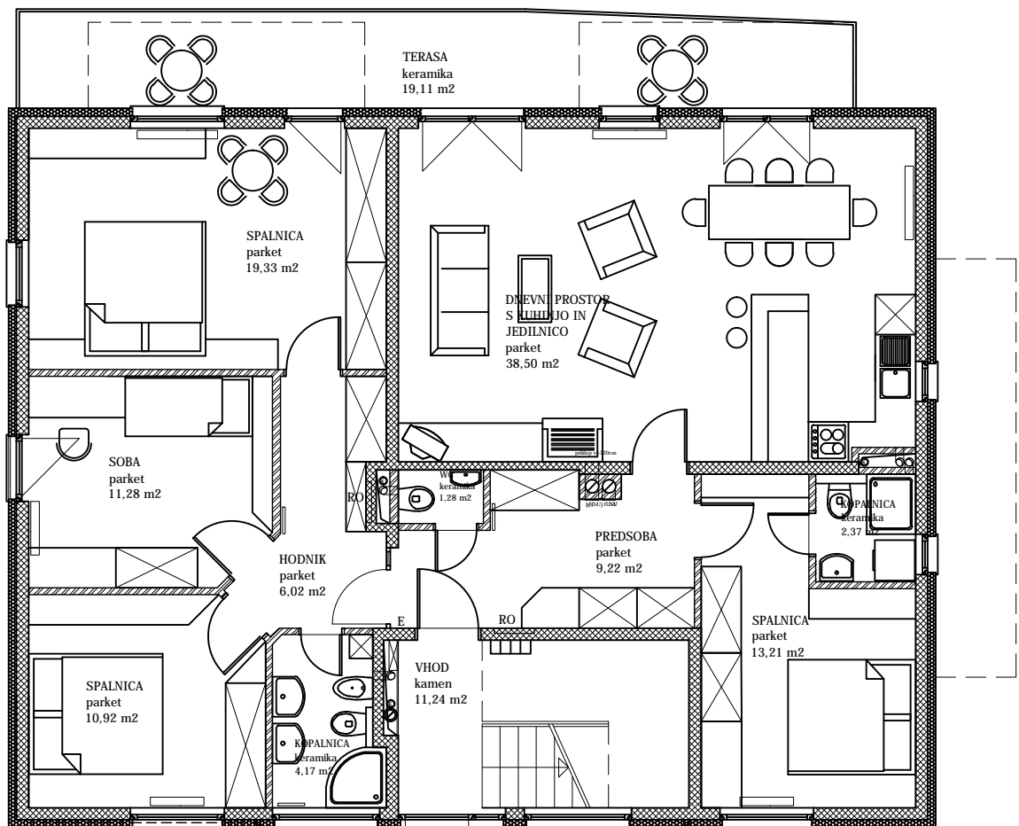
PRITLIČJE objekt B M 1:100
