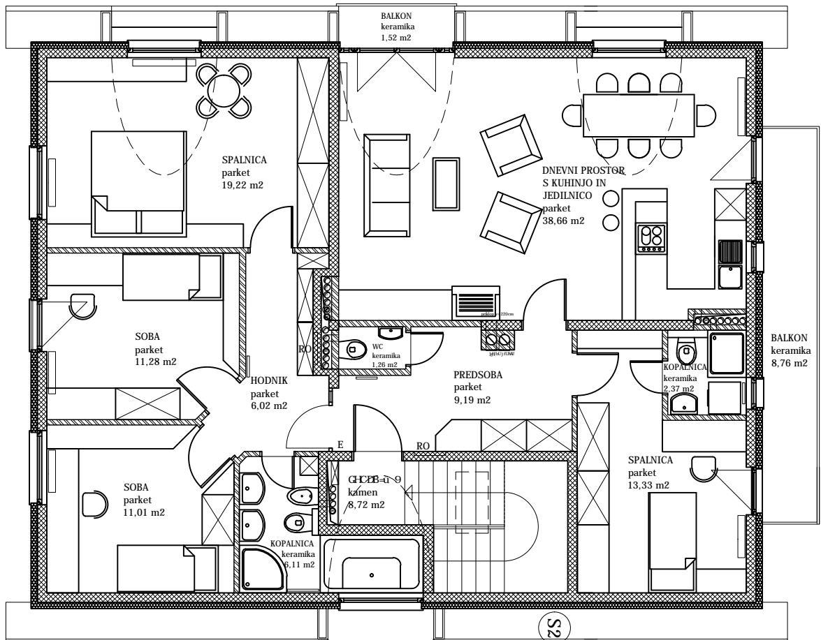
MANSARDA objekt A M 1:100
