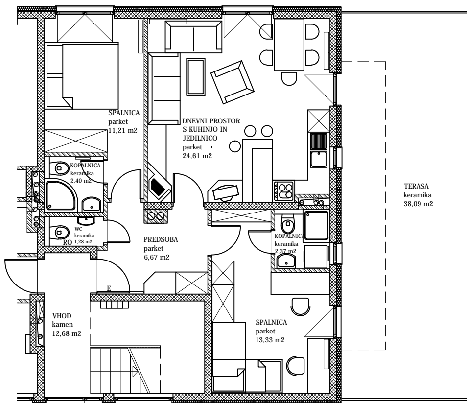
PRITLIČJE objekt A M 1:100
