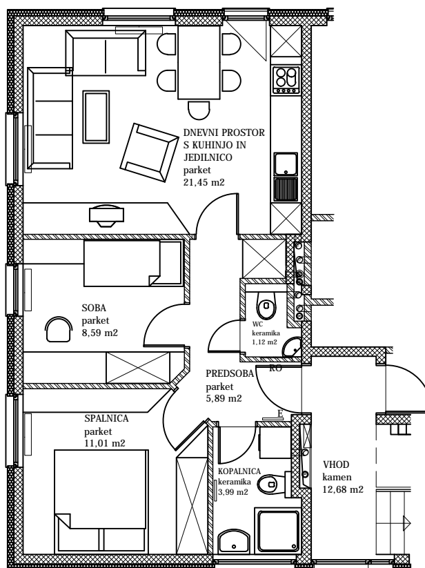
PRITLIČJE objekt A M 1:100
